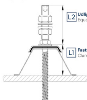
Trapezformet profil og sandwichelement Trapeze profile and sandwich element
