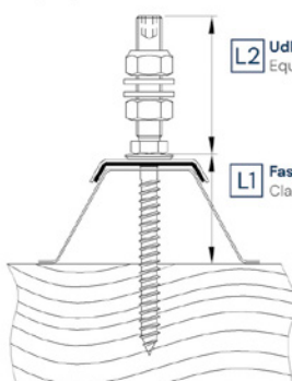
Trapezformet profil og sandwichelement Trapeze profile and sandwich element
