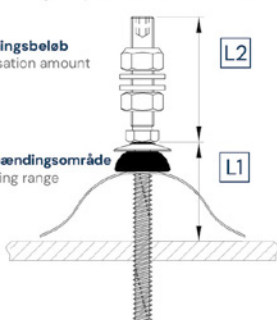
Bølgeprofil og sandwichelement Corrugated profile and sandwich element
