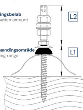
Bølgeprofil og sandwichelement Corrugated profile and sandwich element
