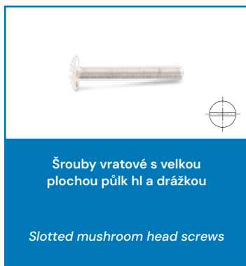
NF E 27-128 Slot A2/A4
