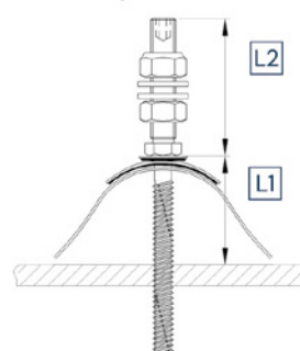
Vlnitý vláknocement Corrugated fibre cement
