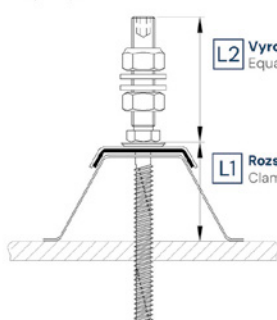
Trapézový profil a sendvičový prvek Trapeze profile and sandwich element
