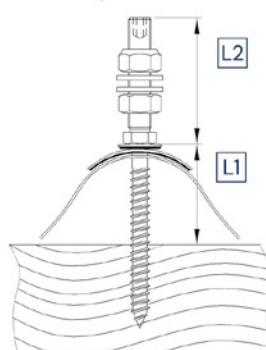
Vlnitý vláknocement Corrugated fibre cement
