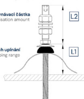
Vlnitý profil a sendvičový prvek Corrugated profile and sandwich element
