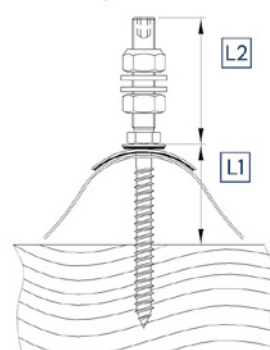
Vlnitý vláknocement Corrugated fibre cement
