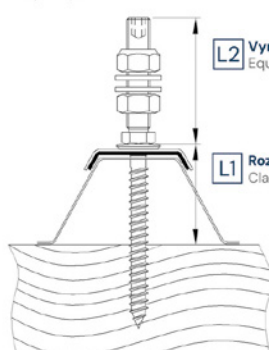
Trapézový profil a sendvičový prvek Trapeze profile and sandwich element
