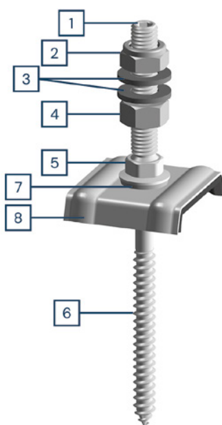
Trapezový profil a sendvičový prvek Trapeze profile and sandwich element
