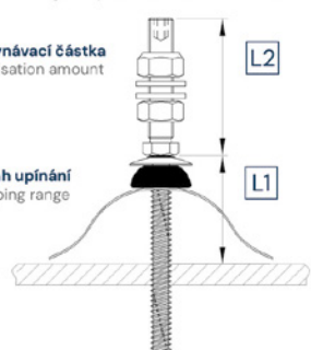
Vlnitý profil a sendvičový prvek Corrugated profile and sandwich element
