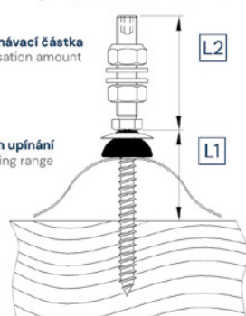
Vlnitý profil a sendvičový prvek Corrugated profile and sandwich element
