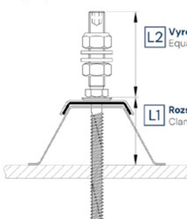
Trapezový profil a sendvičový prvek Trapeze profile and sandwich element
