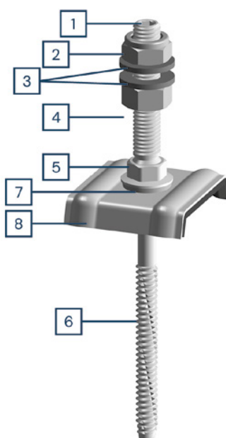
Profil trapézoïdal et élément sandwich Trapeze profile and sandwich element
