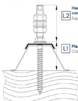
Profil trapézoïdal et élément sandwich Trapeze profile and sandwich element
