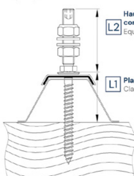
Profil trapézoïdal et élément sandwich Trapeze profile and sandwich element
