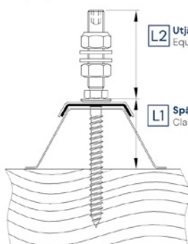
Trapetsformad profil och sandwichelement Trapeze profile and sandwich element
