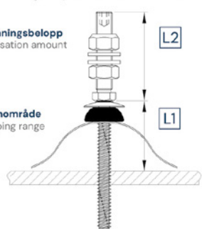
Trapetsformad profil och sandwichelement Trapeze profile and sandwich element
