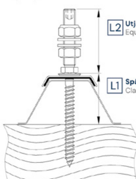
Trapetsformad profil och sandwichelement Korrerad profil och sandwichelement Trapeze profile and sandwich element Corrugated profile and sandwich element
