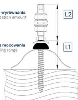
Profil falisty i element warstwowy Corrugated profile and sandwich element
