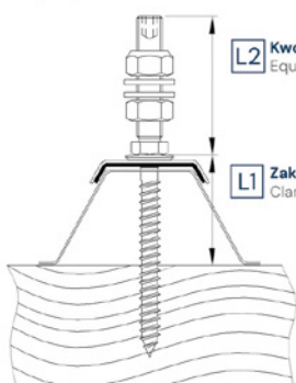
Profil trapezowy i element warstwowy Trapeze profile and sandwich element
