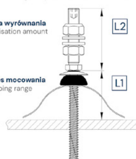
Profil falisty i element warstwowy Corrugated profile and sandwich element
