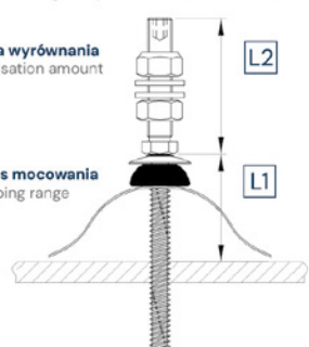
Profil falisty i element warstwowy Corrugated profile and sandwich element
