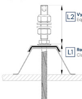
Trapézový profil a sendvičový prvek Trapeze profile and sandwich element
