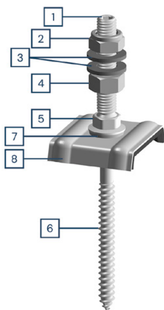
Trapézový profil a sendvičový prvek Trapeze profile and sandwich element
