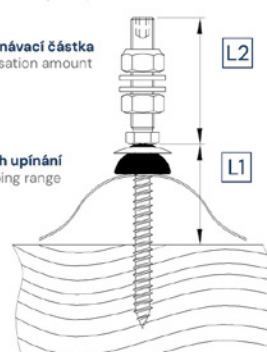
Vlnitý profil a sendvičový prvek Corrugated profile and sandwich element
