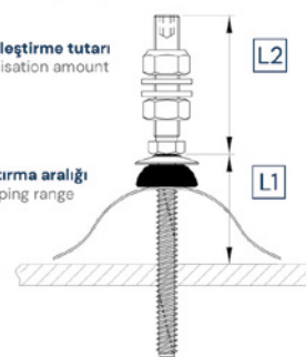
Oluklu profil ve sandviç eleman Corrugated profile and sandwich element
