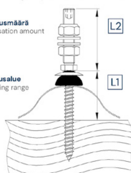
Aaltoprofiili ja sandwich-elementti Corrugated profile and sandwich element
