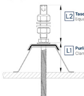
Puolisuunnikkaan muotoinen profiili ja sandwich-elementti Trapeze profile and sandwich element
