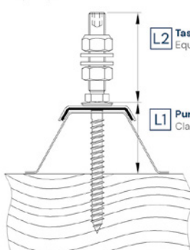
Puolisuunnikkaan muotoinen profiili ja sandwich-elementti Trapeze profile and sandwich element
