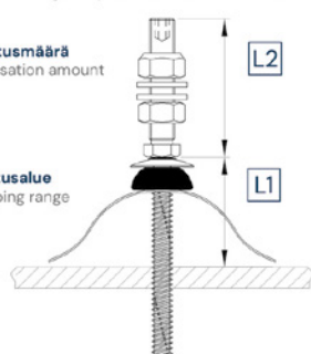
Aaltoprofiili ja sandwich-elementti Corrugated profile and sandwich element
